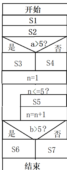
N-S图
